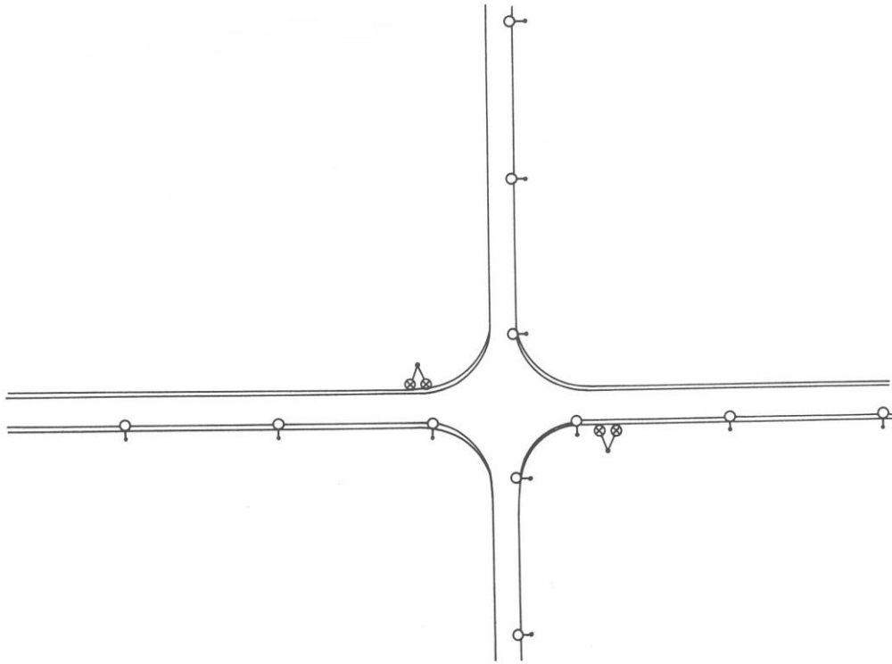
Figur 40: Stolpplacering i enkel okanaliserad fyrvägskorsning: antingen stolpar eller högmastar. Bild: REBEL 91.
