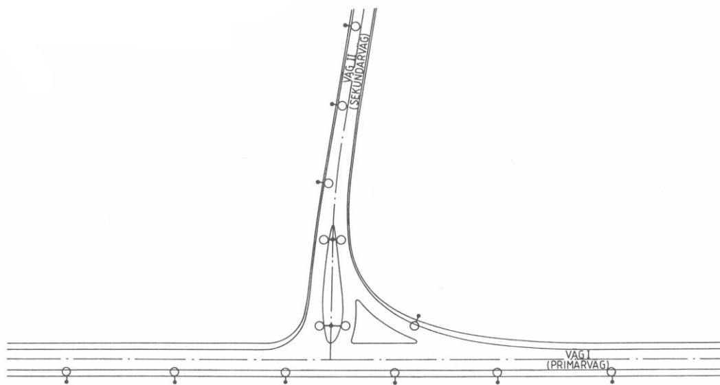
Figur 46: I kanaliserade korsningar med stora refuger kan dessa ibland utnyttjas för stolpplacering. Bild: REBEL 91.
