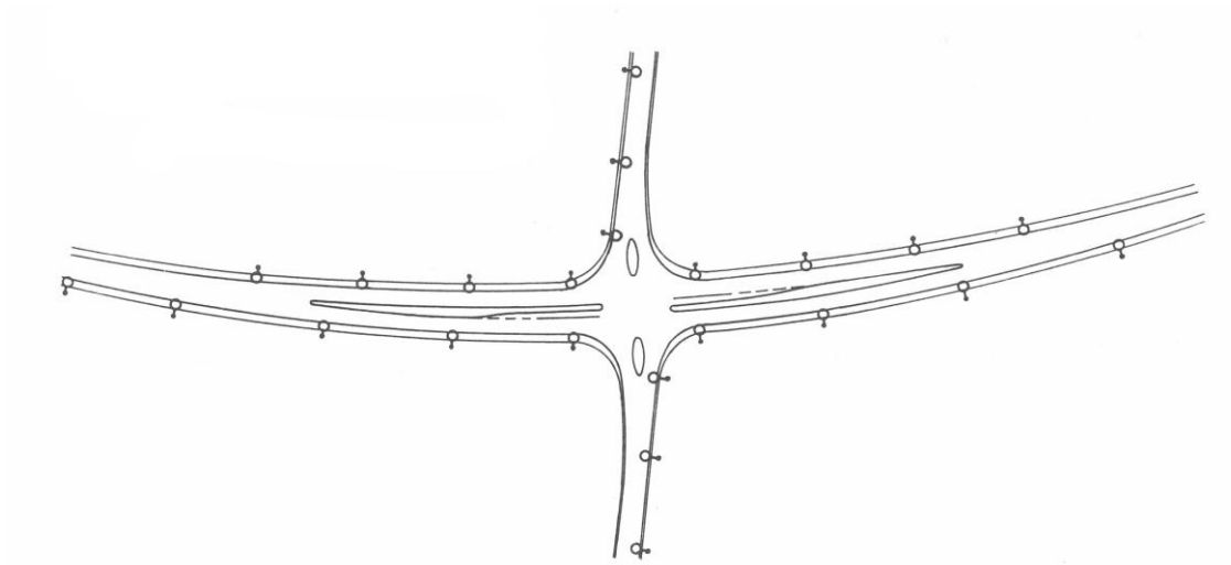
Figur 45: Stolpplacering i fyrvägskorsning med breddad sektion. Enkelsidig placering kan övergå i sicksackplacering och därefter dubbelsidig placering. Bild: REBEL 91.
