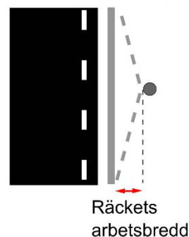
Figur 12: Vänster: Eftergivliga stolpar ska placeras på ett avstånd \geq d_e från körbanekant, enligt Tabell 3, och om möjligt minst 0,5 m från beläggningskant. Mitten: Oeftergivliga stolpar ska placeras utanför säkerhetszonen. Höger: Om vägen har räcken ska stolpar placeras bakom räcke och utanför räckes arbetsbredd.
